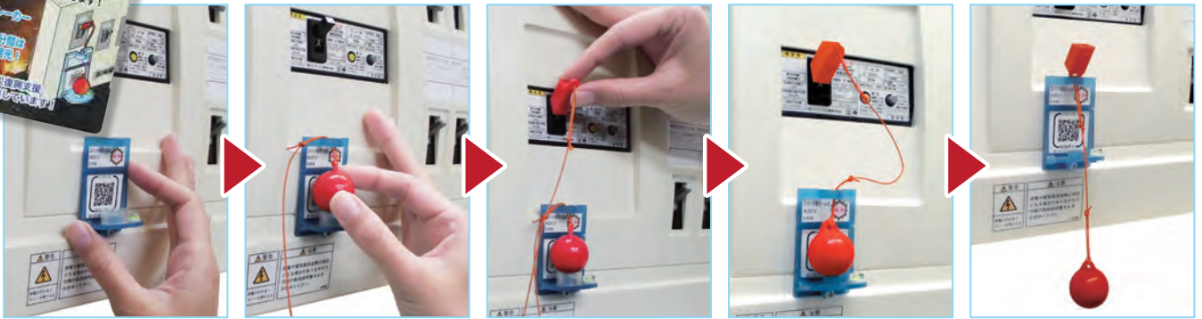
本体の水平計を見てブレーカーに取り付けます
